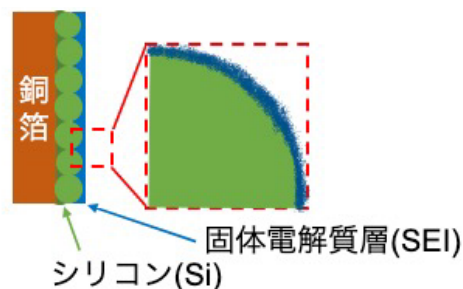
図. 人工 SEI 皮膜を形成した Si 電極
